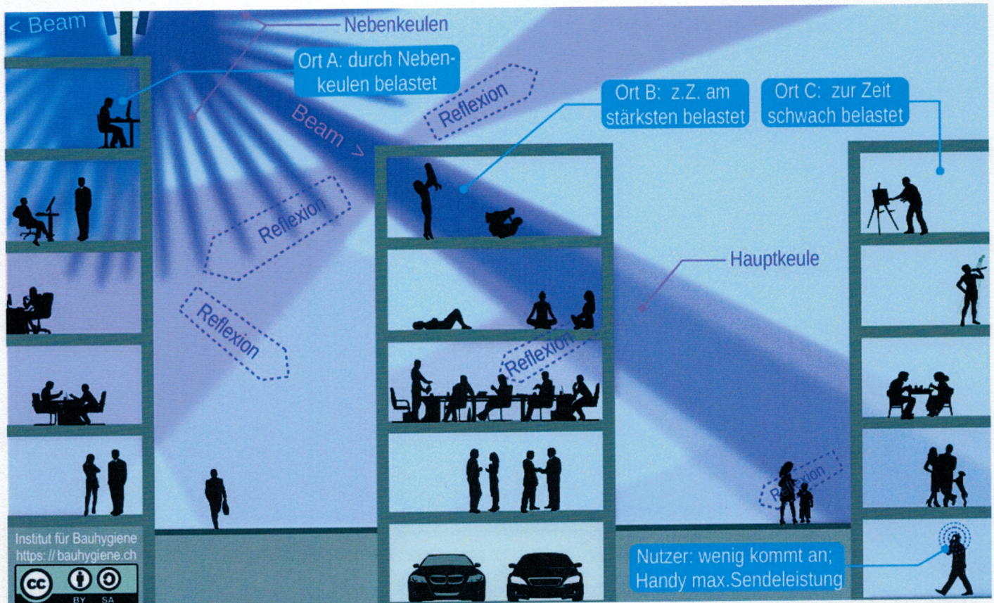
Beam (Strahlenkeule) einer mMIMO-Antenne. Es sind pro Antenne zeitgleich bis zu 8 Beams möglich, die inert Millisekunden laufend ihre Richtung ändern. Auf dem Weg zum Ziel wird der Beam z. T. absorbiert, er durchdringt z. T. Bauteile und wird z. T. an diesen reflektiert/gestreut. Dabei werden Orte unterschiedlich belastet, direkt und indirekt (Reflexion). In der Praxis ist die Strahlungsausbreitung viel komplexer und die Exposition viel heterogener, als in dieser vereinfachten Grafik darstellbar. Nicht zuletzt deshalb sind Messungen und Simulationen mit grossen Unsicherheiten behaftet.
